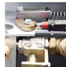
Sicherheitsabschaltung Domsieb im Innenraum
